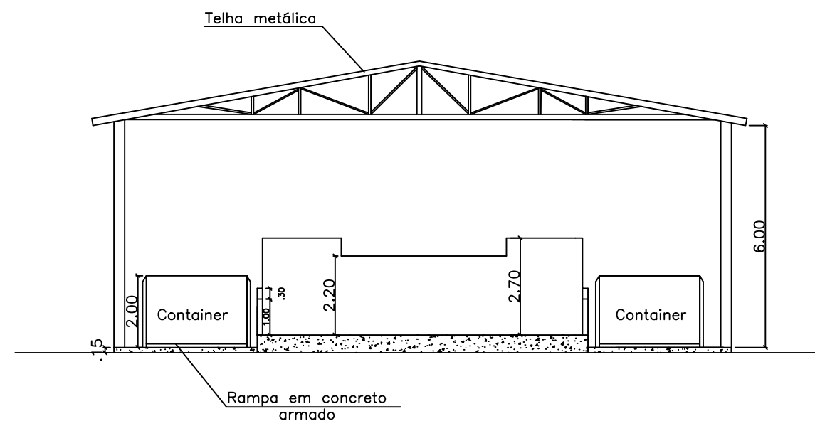
3 Corte BB 1:150
