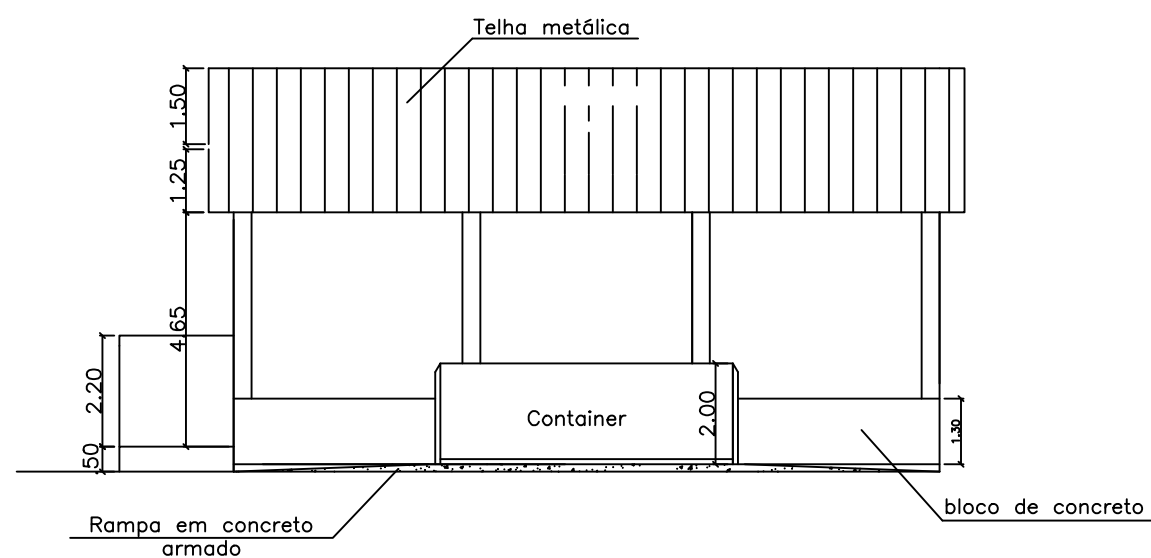
2 Corte AA 1:150
