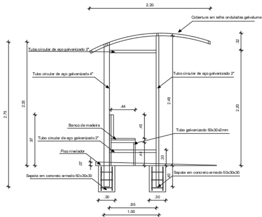
Figura 2 - Corte Lateral
