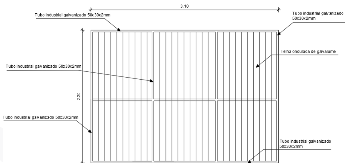
Figura 3 - cobertura
