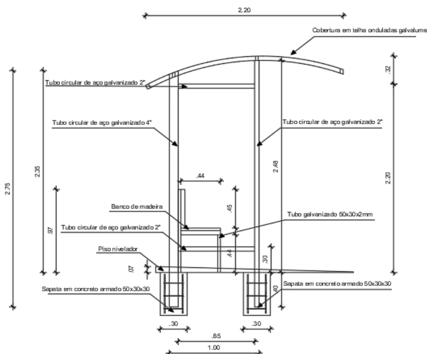
Figura 2 - Corte Lateral
