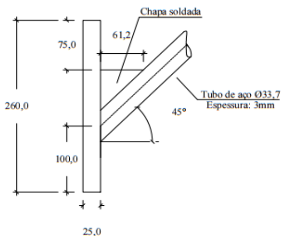
③ Ligação Braço-Sapata Escala 1:5
