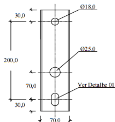
② Sapata - Detalhe Furação Escala 1:5
