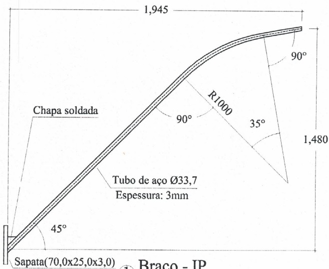
① Braço - IP Escala 1:25
