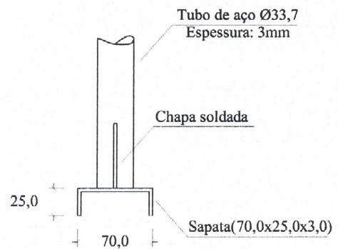
④ Vista Superior Escala 1:5
