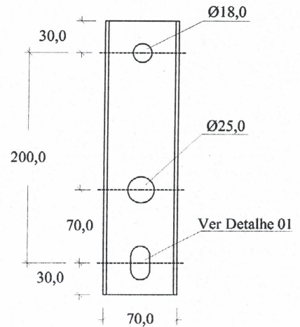
② Sapata - Detalhe Furação Escala 1:5
