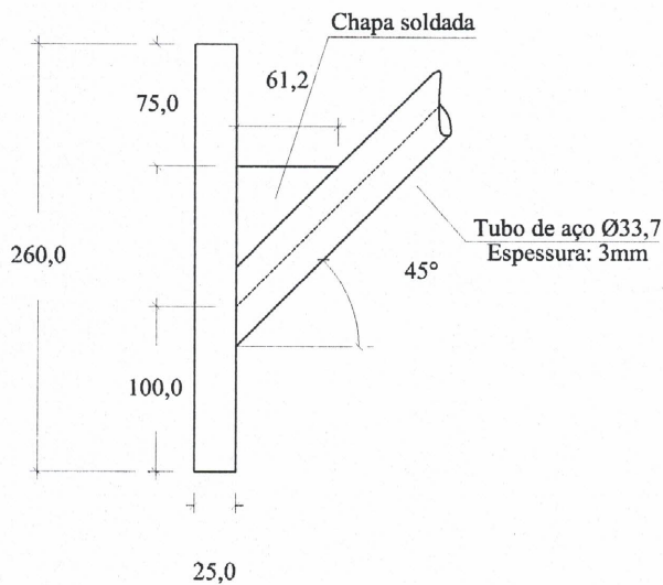
③ Ligação Braço-Sapata Escala 1:5
